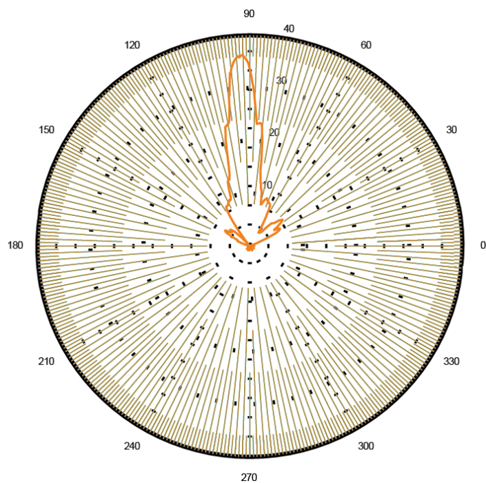
H-Plane Pattern (QAD 1137 - 90 SD HP)
