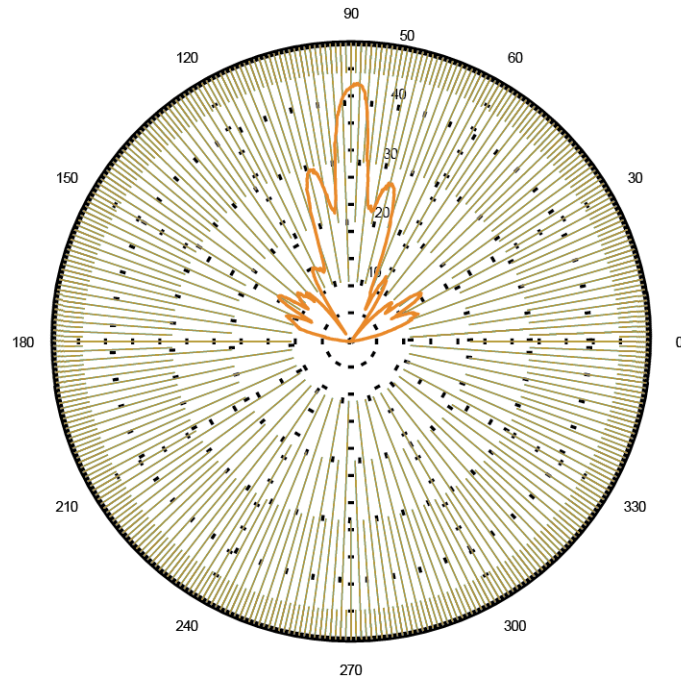
E-Plane Pattern (QAD 1137 - 90 SD HP)
