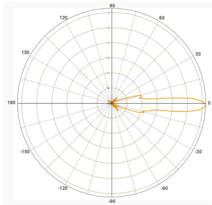
E-Plane Pattern (QAD 0631 - 75 SD)
