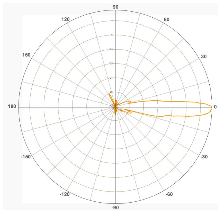
H-Plane Pattern (QAD 0631 - 75 SD)
